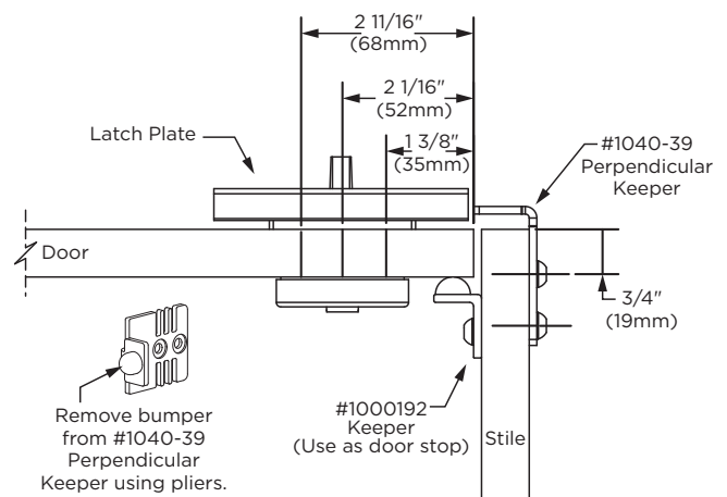
Fig. 11e: Perpendicular/Alcove Inswing
