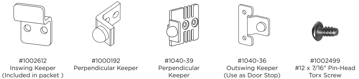
Fig. 9d: Inline Inswing
