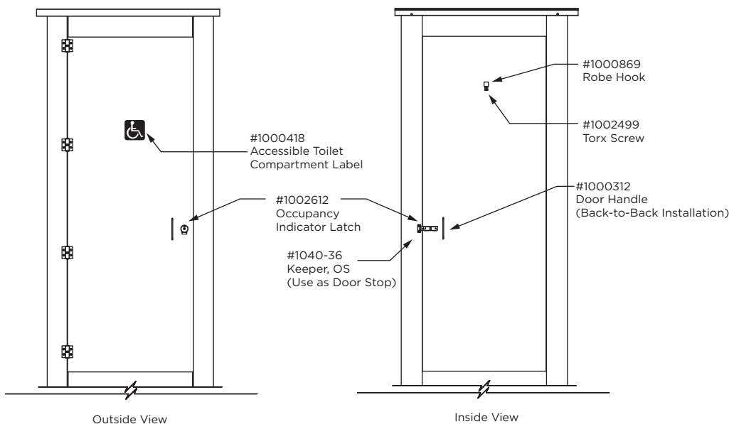
Fig. 12b: Outswing Door
