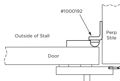
Fig. 11d: Perpendicular/Inswing Door
